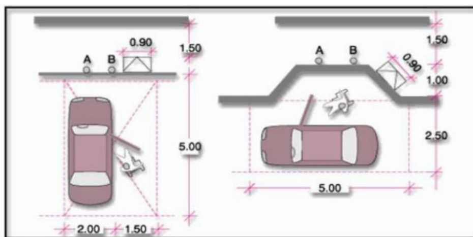
Εικόνα 6: Διαμόρφωση θέσης στάθμευσης ΑμεΑ
