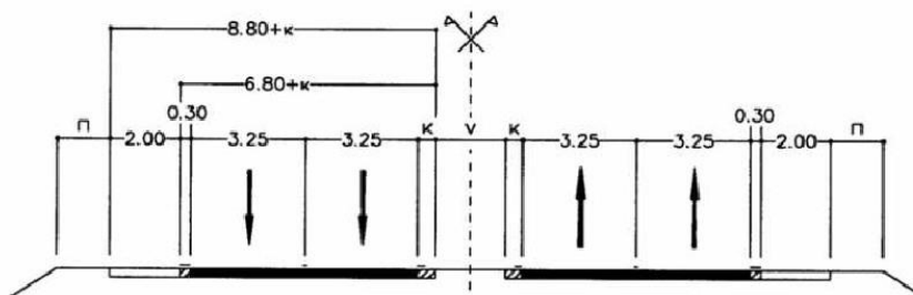
Τυπική διατομή γ4νσ - κλάδος με 2 λωρίδες ανά κατεύθυνση και διαχωριστική νησίδα πλησίον της πρόσβασης στον κυκλικό κόμβο
