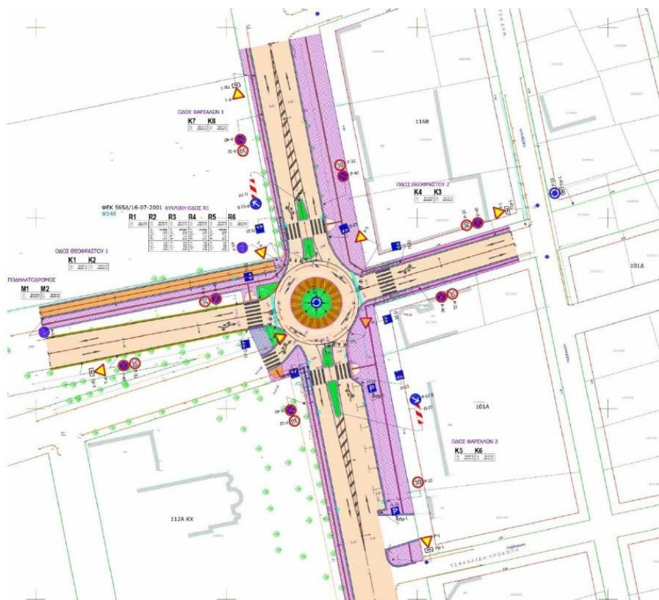
Εικόνα 6. Οριζοντιογραφική αποτύπωση Κ3 (Ιδία επεξεργασία)
