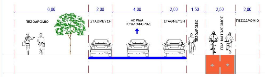
Τυπική διατομή οδού Αγ. Τριάδος τυπική διατομή ΔΤ_6
