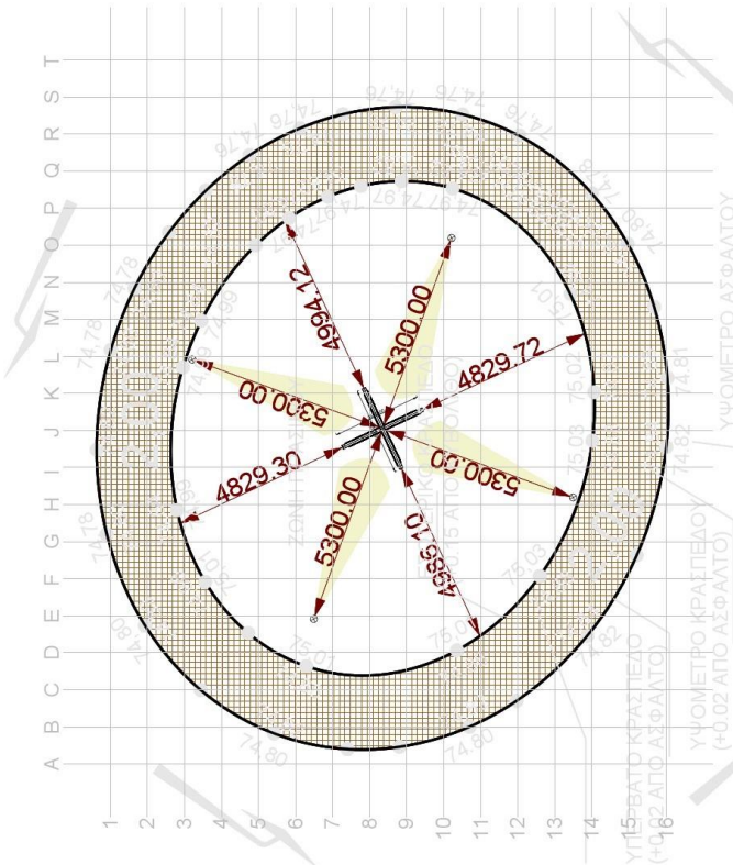
ΚΑΤΟΥΗ - ΔΙΑΓΡΑΜΜΑ ΦΩΤΙΣΜΟΥ
