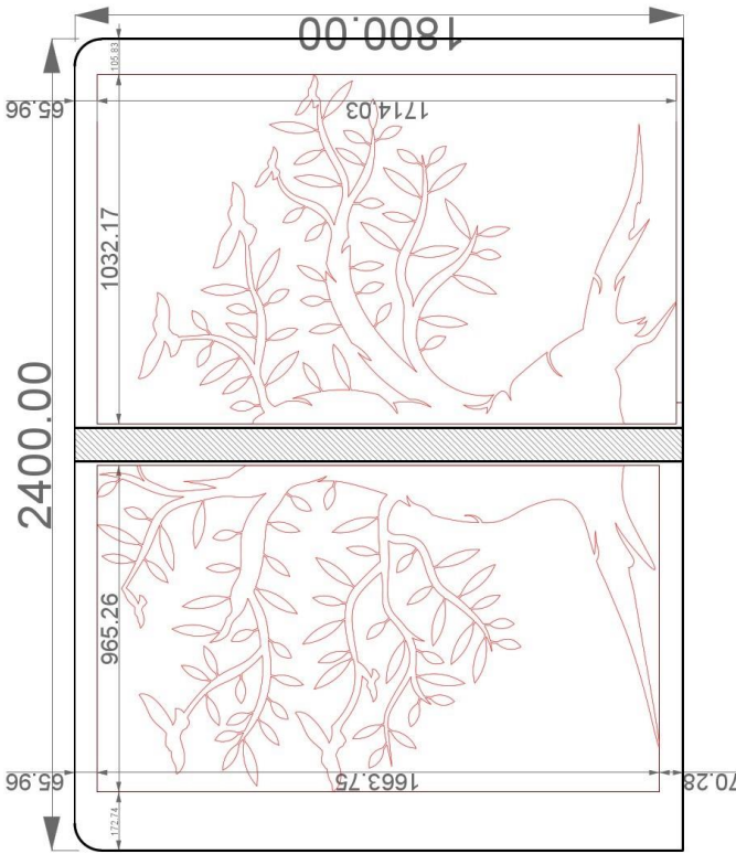
ΜΕΤΑΛΛΙΚΗ ΠΛΑΚΑ ΣΤΟ ΣΧΗΜΑ ΤΗΣ ΕΛΙΑΣ
