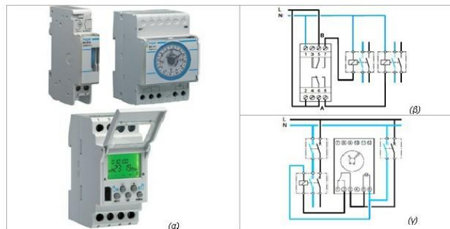
Χρονοδιακόπτες: (α) ηλεκτρομηχανικοί (άνω) και ηλεκτρονικός (κάτω), (β) Παράδειγμα συνδεσμολογίας ελέγχου δύο ηλεκτρονόμων από ένα χρονοδιακόπτη, (γ) Παράδειγμα συνδεσμολογίας ελέγχου δύο κυκλωμάτων φωτισμού από ένα χρονοδιακόπτη
