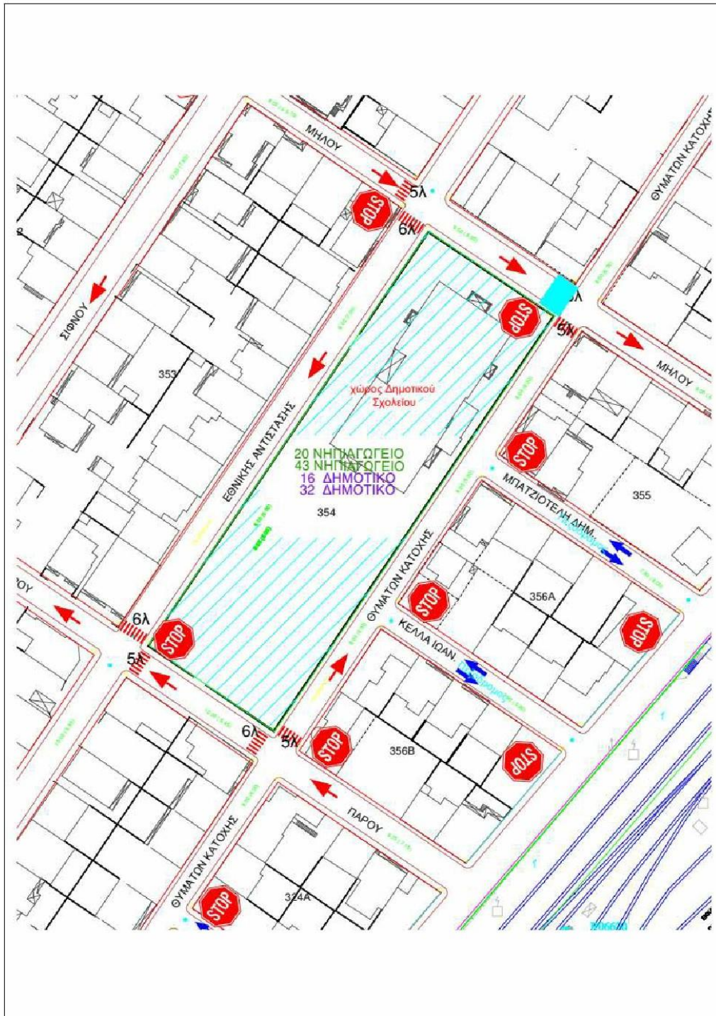
ΣΧΕΔΙΟ 2: ΟΡΙΖΟΝΤΙΟΓΡΑΦΙΑ ΔΙΑΒΑΣΗΣ ΕΠΙ ΤΗΣ ΟΔΟΥ ΜΗΛΟΥ
