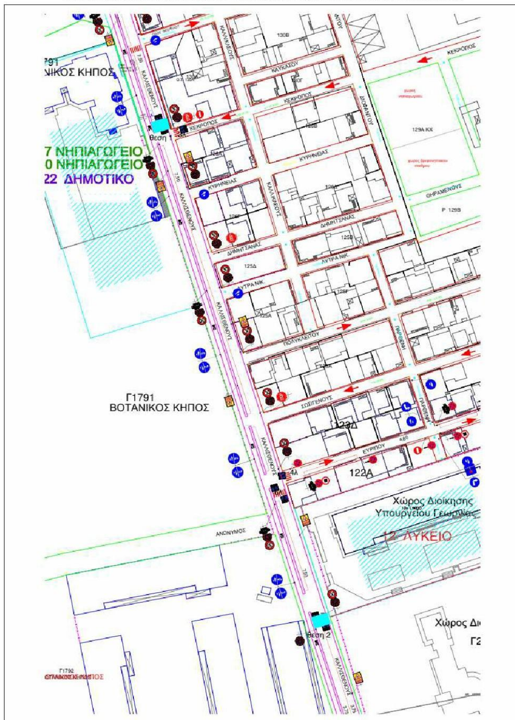
ΣΧΕΔΙΟ 8: ΟΡΙΖΟΝΤΙΟΓΡΑΦΙΑ ΔΙΑΒΑΣΕΩΝ ΕΠΙ ΤΗΣ ΟΔΟΥ ΚΑΛΛΙΣΘΕΝΟΥΣ ΣΤΟ ΥΨΟΣ ΤΗΣ ΟΔΟΥ ΚΕΚΡΟΠΟΣ ΚΑΙ ΑΠΕΝΑΝΤΙ ΑΠΟ ΤΗΝ ΑΠΟΚΕΝΤΡΩΜΕΝΗ ΔΙΕΥΘΥΝΣΗ ΘΕΣΣΑΛΙΑΣ
