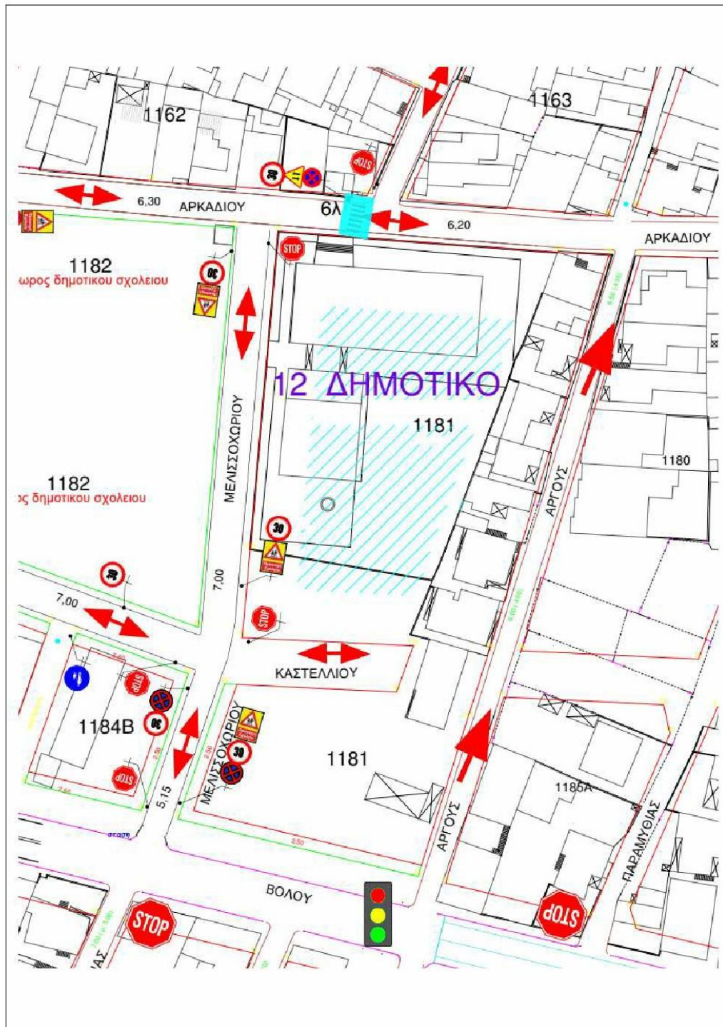
ΣΧΕΔΙΟ 18: ΟΡΙΖΟΝΤΙΟΓΡΑΦΙΑ ΔΙΑΒΑΣΗΣ ΕΠΙ ΤΗΣ ΟΔΟΥ ΑΡΚΑΔΙΑΣ
