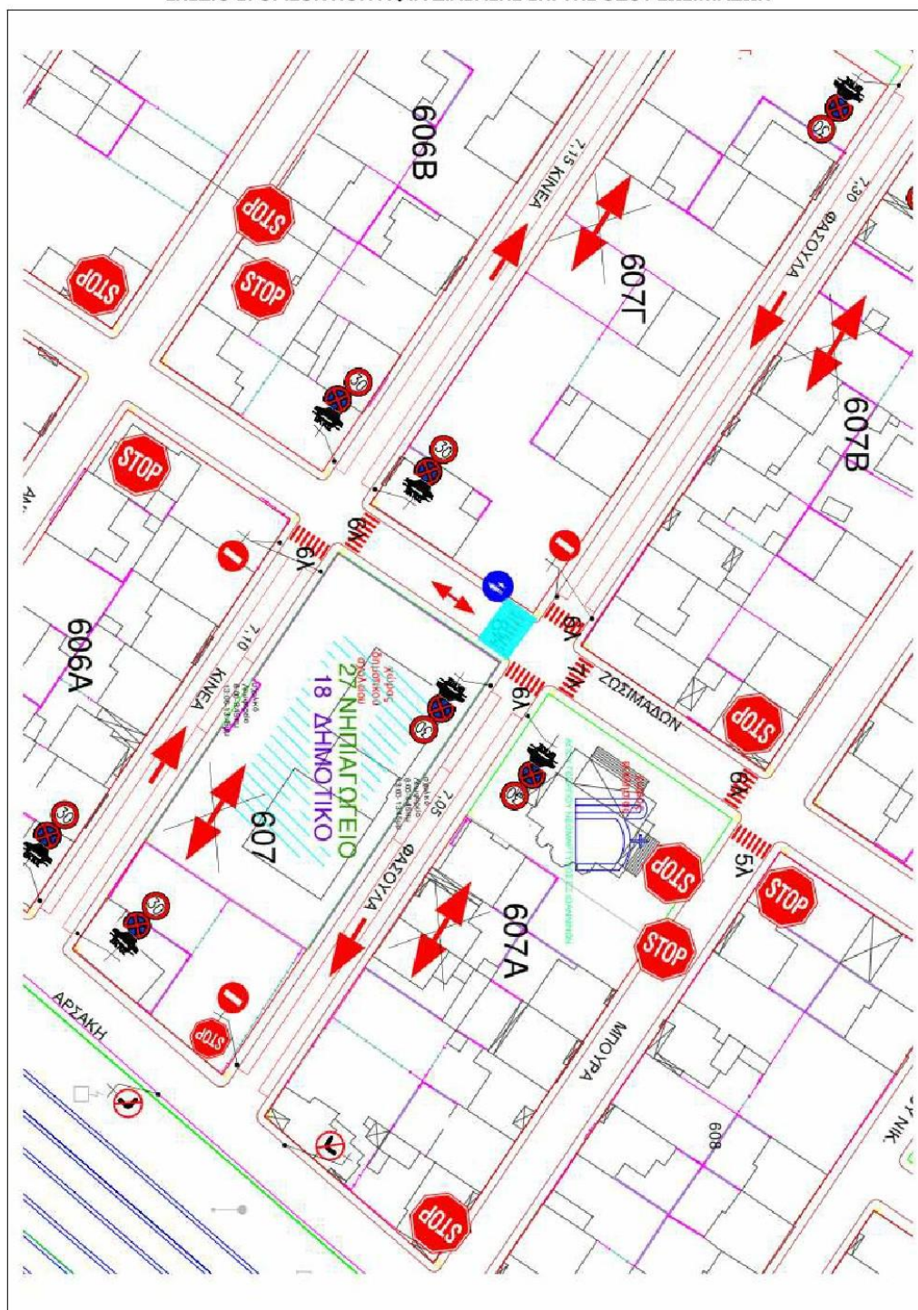
ΣΧΕΔΙΟ 1: ΟΡΙΖΟΝΤΙΟΓΡΑΦΙΑ ΔΙΑΒΑΣΗΣ ΕΠΙ ΤΗΣ ΟΔΟΥ ΖΩΣΙΜΑΔΩΝ
