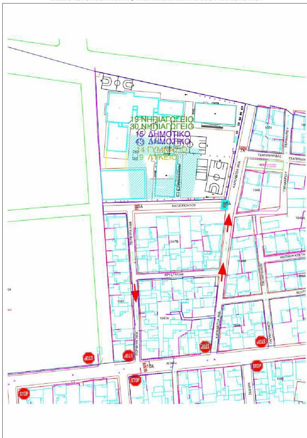
ΣΧΕΔΙΟ 19: ΟΡΙΖΟΝΤΙΟΓΡΑΦΙΑ ΔΙΑΒΑΣΗΣ ΕΠΙ ΤΗΣ ΟΔΟΥ ΧΑΤΖΟΠΟΥΛΟΥ
